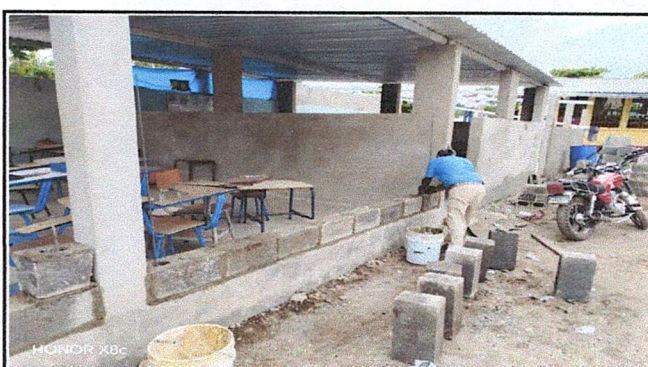
Foto 4: Suministro de block para muro (incluye columnas de 0.15 x 0.15 x 1.00 mts con hierro Ø 1/2" est. 1/4 + solera de 0.20 x 0.15 con hierro Ø 3/8" est. 1/4")
