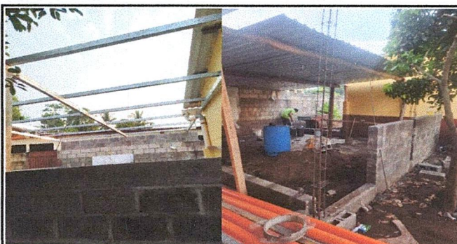
Foto 5: Sustrucción de costanera de madera por costanera metálica 2 x 3, Sustrucción de lámina por lámina troquelada cal. 26
