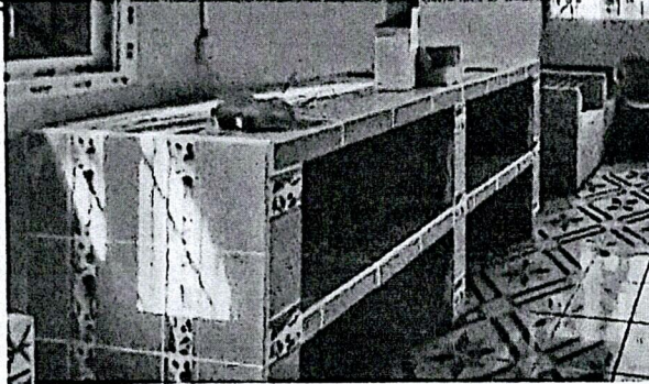
Foto 1: Se realizara el suministro de mueble de cocina de concreto mas revestimiento de azulejos de 3.00X0.85X0.80 mts
