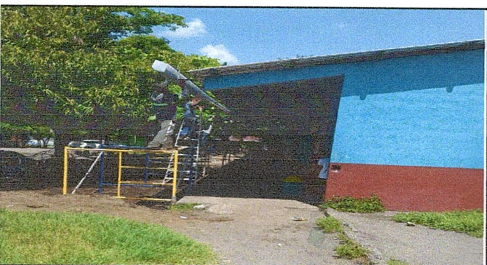
Foto 5: Instalación de canales de metal y bajadas de agua plubial tubo pvc modulo 1 consta de 3 aulas, adelante y atrás
