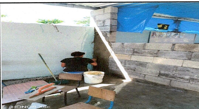
Foto 3: suministro de repello . Modulo aula. Suministro e instalación de balcón metálico con marco de angular 1" x 1" reforzado con hierro 3/8" (incluye pago de mano de obra)
