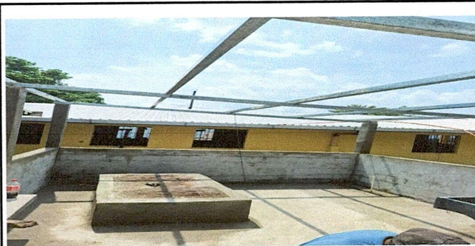
Foto 4: Sustitución de costanera de madera por costanera metálica 2 x 3. Sustitución de lámina por lámina troquelada cal. 26
