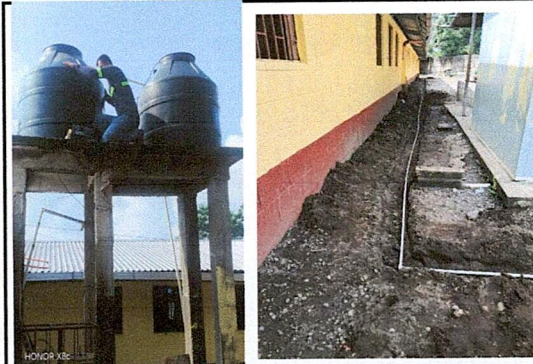
Foto 6: Sustitución de tinaco por tinaco de agua 1,100 lts. Suministro de tubería Ø 1" mas accesorios (instalación para servicios sanitarios)
