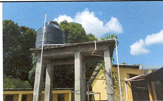
Foto 6: Sustitución de tinaco por tinaco de agua 1,100 lts. Suministro de tubería Ø 1" mas accesorios (instalación para servicios sanitarios)
