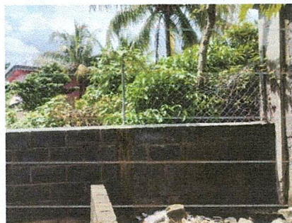
4. Suministro de block para circulación de muro perimetral (incluye columnas de 0.15 x 0.15 x 1.00 mt con hierro Ø 1/2" est. 1/4 + solera de 0.20 x 0.15 con hierro Ø 3/8" est. 1/4")
