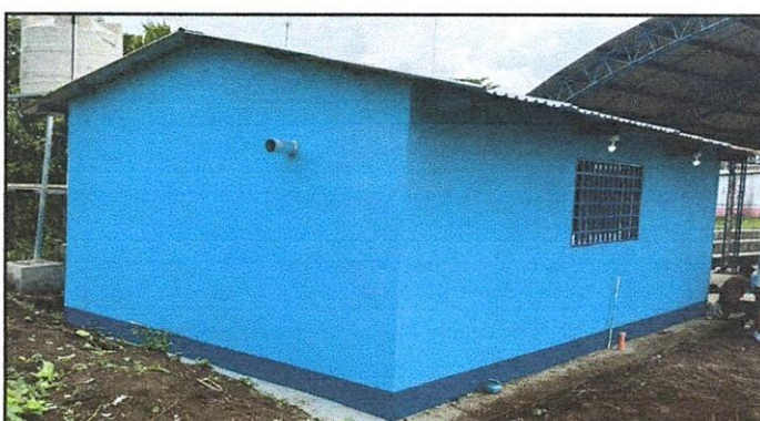
FOTO 4: Aplicación de repello y cernido en muros de cocina interior y exterior
