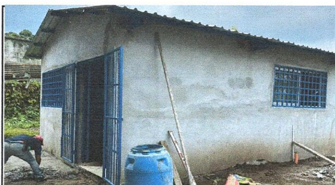
FOTO 4: Apliación de repello y cernido en muros de cocina interior y exterior
