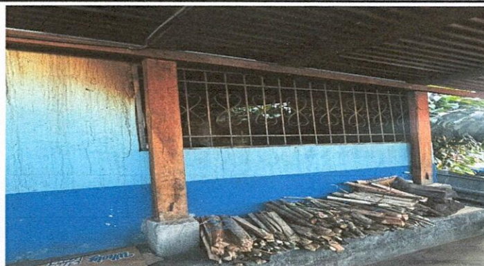
Foto1: Sustitución de cubierta de lamina troquela calibre 26
