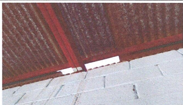
FOTO 3: Mantenimiento de estructura portante de metal
