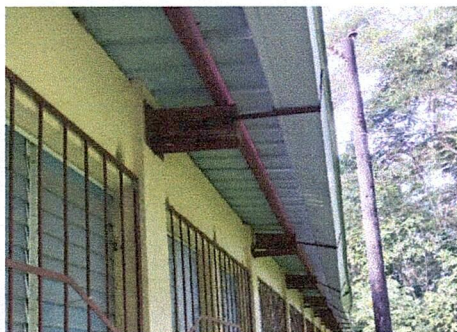
Foto 3: Mantenimiento de canal de metal + bajadas de agua pluvial pvc 3"
