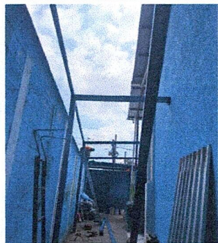
Foto 13: Suministro de lámina troquelada calibre 26+ estructura de soporte de metal (en áreas de pasillos, ingreso principal y patio)
