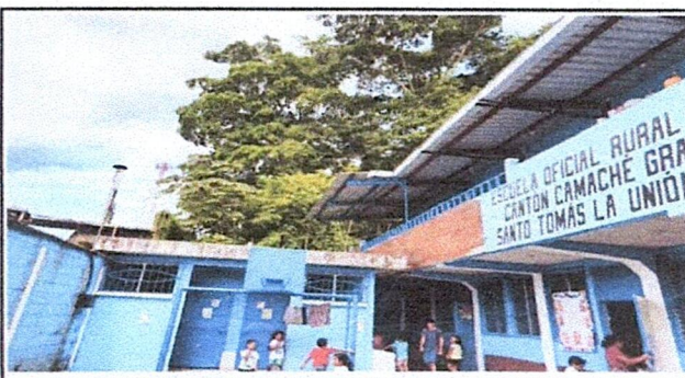
Foto 6: Suministro de canal de metal + bajadas de agua pluvial pvc 3"
