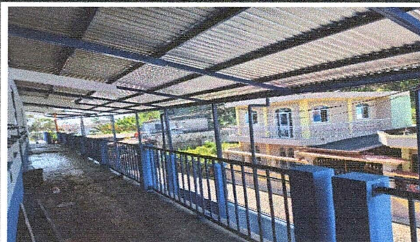
Foto2: Suministro de 98 metros cuadrados de lámina troquelada calibre 26, más estructura de metal, en área de pasillo, ingreso y egreso del establecimiento.
