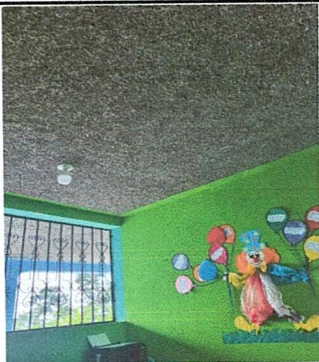
Foto 5: Reparación de sistema eléctrico de iluminación y fuerza (tomacorrientes, plataformas, focos, interruptores, 2 tableros, cableado y entubado)
