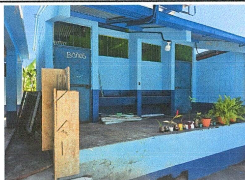
Foto 4: Mantenimiento de puerta de metal de 1.00 x 2.20 (lijado, cepillado y aplicación de 2 manos de pintura anticorrosiva)
