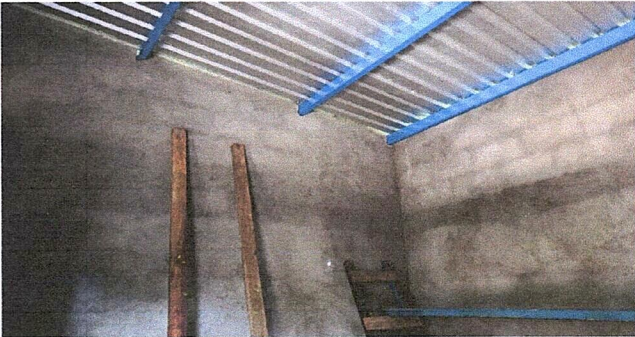
Foto 2: Sustitución de lámina, por lámina troquelada aluzinc calibre 26 + sustitución de estructura portante de metal
