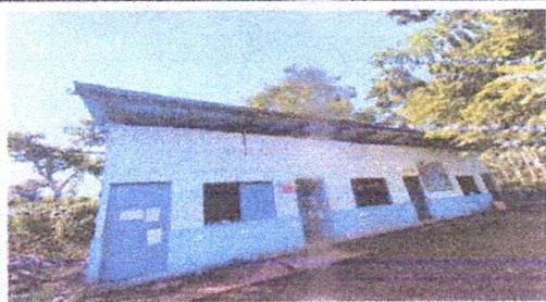
Foto 5: Sustitución de lámina, por lámina troquelada aluzinc calibre 26 + sustitución de estructura portante de metal (techado de lámina y área posterior de aulas)
