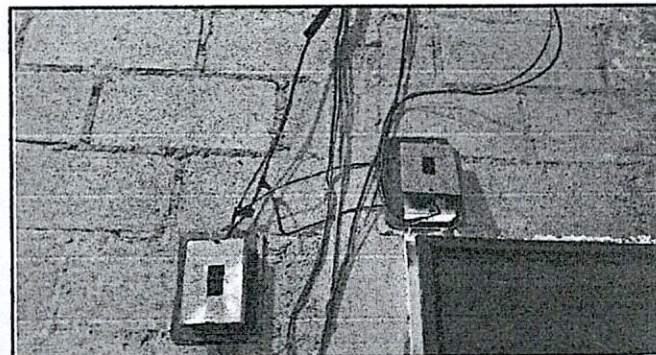
Foto 4: Reparación de sistema eléctrico instalación de tablero de 4 circuitos + dados de filipon y unidades de luminarias.
