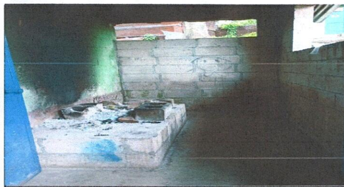
Foto 5: SE REALIZARA LA SUSTITUCIÓN DE ESTUFA RURAL POR ESTUFA RURAL DE LADRILLO CON CHIMENEA DE CONCRETO MAS PLANCHA Y PARRILLA DE METAL
