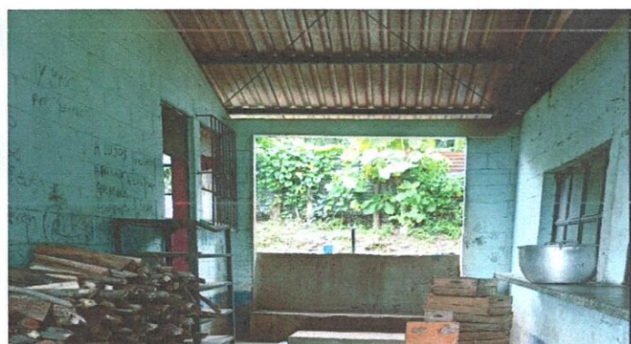
Foto 4: SE REALIZARA EL SUNISTRO DE MUEBLE DE COCINA DE CONCRETO
