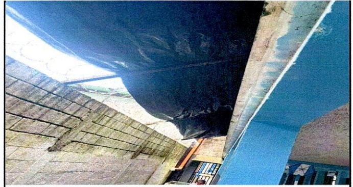
Foto 2: Suministro de estructura de techo y cubierta de lámina para mejorar voladizo de aulas hacia patiosuministro de bajadas de agua pluvial con tubo de 3" Ø
