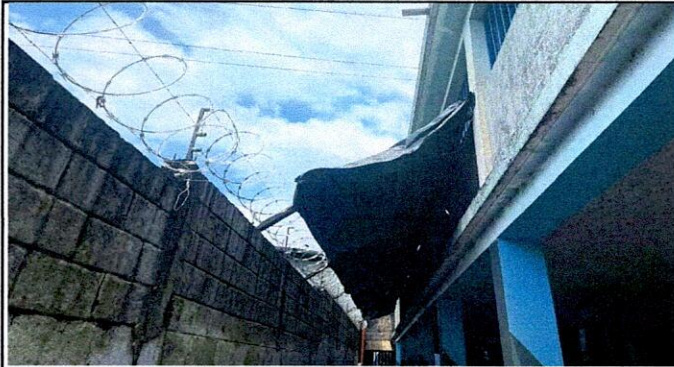
Foto 1: Suministro de estructura de techo y cubierta de lámina para mejorar voladizo de aulas hacia patio y se realizará el suministro de canales de agua pluvial de metal + sujeciones
