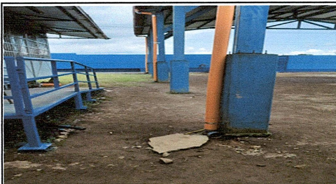
Foto 2: Reparación de bajada de agua pluvial, tubo PVC 4".
