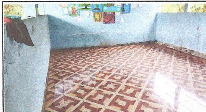
Foto 6: SUSTITUCIÓN DE PISO DE TORTA DE CEMENTO POR PISO CERAMICO EN AULA DE SEGUNDO NIVEL
