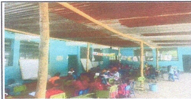
Foto 5: Instalación de Columnas de 20 cm x 25 cm x 4.40
