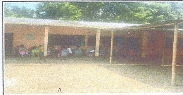
Foto 6: Instalación de Columnas de 20 cm x 25 cm x 4.40
