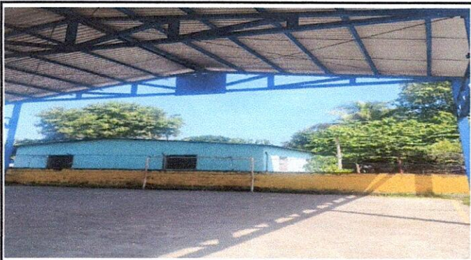
Foto 3: Suministro de electromalla con tubo galvanizado
