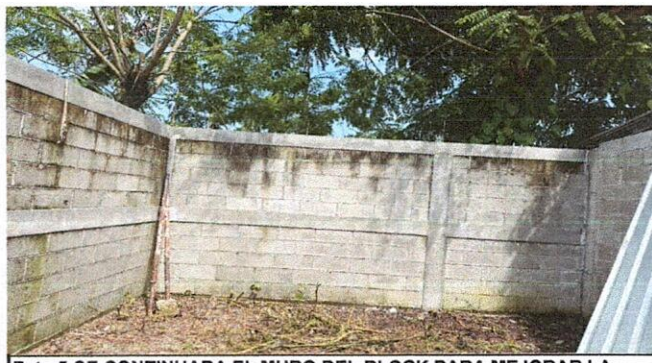
Foto 5: SE CONTINUARA EL MURO DEL BLOCK PARA MEJORAR LA ALTURA DE COCINA
