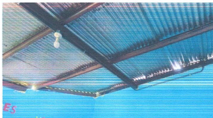
Foto 4: SE REALIZARA EL MANTENIMIENTO A ESTRUCTURA DE SOPORTE DE CUBIERTA
