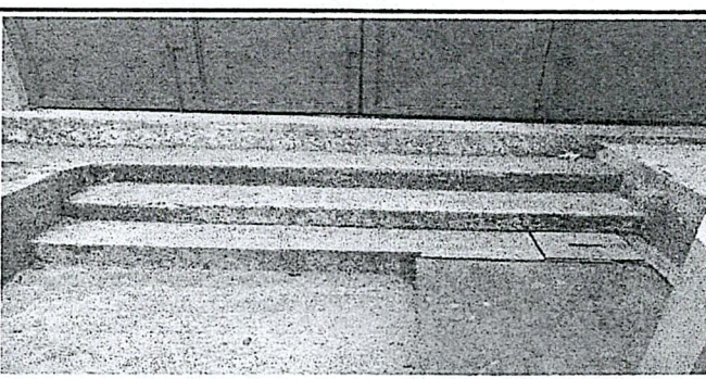
Foto 6: Sustrucción de gradas por rampa de concreto
