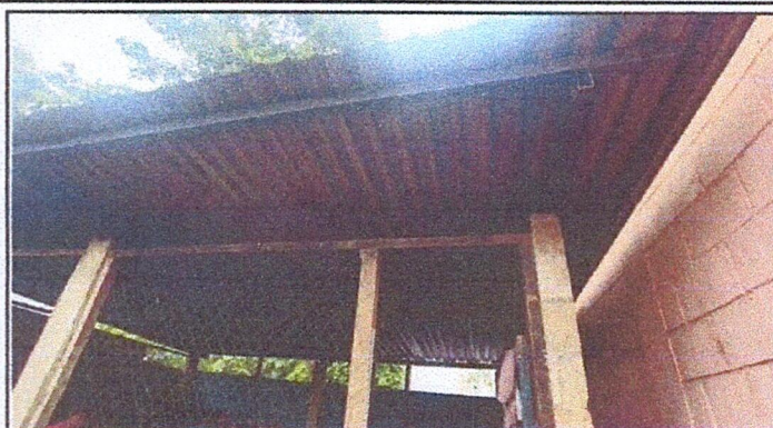
Foto 2: sustitución de estructura de soporte y sustitucion de lamina troquelada
