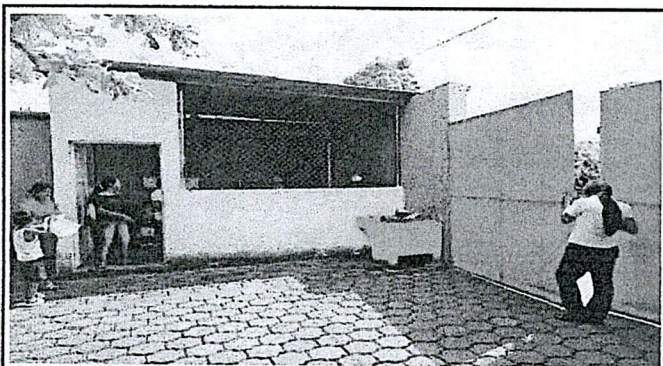
Foto 3: Referencia renglón 1.4, 1.5 y 1.9 (suministro de balcon de metal, ventana de pvc. + estructura metalica para cubrir vano de ventana).
