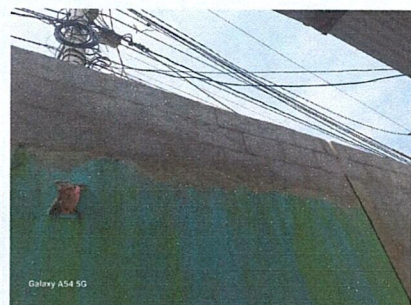
Foto 5: Suministro de block para circulación de muro perimetral (incluye columnas de 0.15 x 0.15 x 0.75 mts con hierro Ø 1/2" est. 1/4 + solera de 0.20 x 0.15 con hierro Ø 3/8" est. 1/4")
