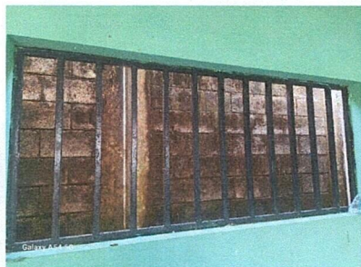
Foto1: Suministro e instalación de balcón metálico con marco de angular 1" x 1" x 1/8" reforzado con hierro 1/2"
