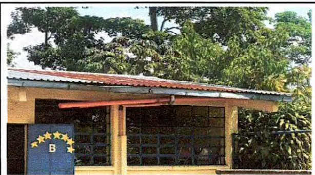
Foto 10: Sustitución de lámina, por lámina troquelada aluzinc calibre 26 y capote en aula No.5 (módulo 2)
