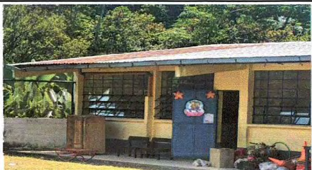
Foto 3: Sustitución de lámina, por lámina troquelada aluzinc calibre 26 y capote en aula No.4 (módulo 1)
