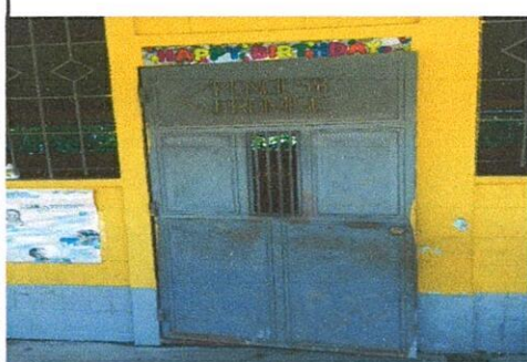
Foto 5: Mantenimiento de puerta de ingreso de 0.91 m x 2.60 m, incluye (Colocación de chapa Yale, lijarse, cepillar y aplicar dos manos de pintura anticorrosiva)
