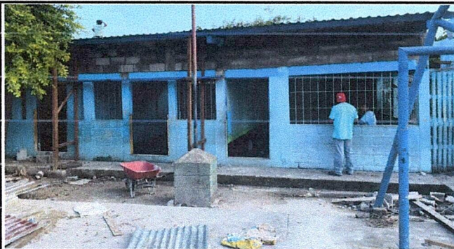
SUSTITUCION DE CUBIERTA DE LAMINA POR LAMINA TROQUELADA CALIBRE
