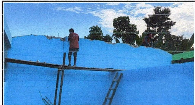
NIVELACION CON LEVANTAMIENTO DE MURO PARA LA PENDIENTE DEL TECHO
