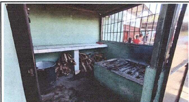
Foto1: Sustitución de estufa rural (completa) incluye chimenea y plancha de metal, mantenimiento de cubierta y estructura de soporte de metal, aplicación de pintura en muros interiores y exteriores.
