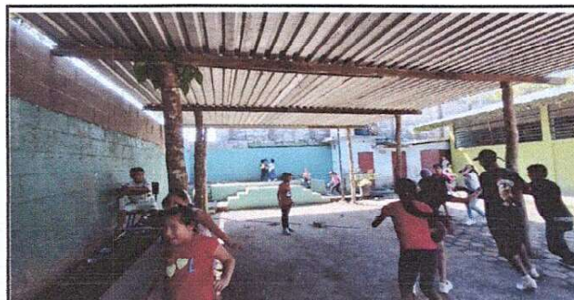
Foto 6: Sustitución de lámina, por lámina troquelada aluzinc calibre 26 Sustitución de estructura de soporte de madera, por metal.
