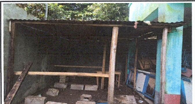
FOTO 3: Sustrucción de estructura de techo y cubierta de lámina
