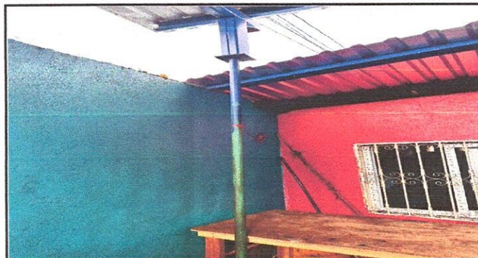
Foto 3 Renglón 1.3: Suministro de columna de concreto de 0.30x0.30x1.20 de alto y suministro de paral de costanera de 4x2 encuachado de 2.70
