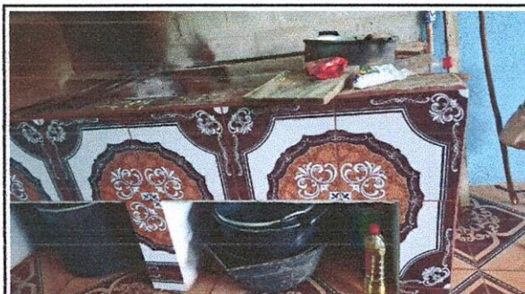
FOTO 4: SUMINISTRO DE CHIMENEA DE CONCRETO+ CAMPANA DE CONCRETO AEREA + REPELLO
