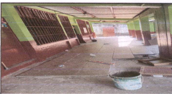
Foto 6: Sustitución de piso de torta de cemento, por piso cerámico en modulo de aulas y corredor
