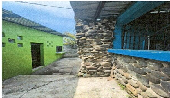
Foto 2: REPARACIÓN DE MURO DE PIEDRA
