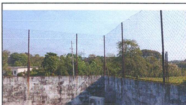
Foto 4: Reparación de muro perimetral, con tubo galvanizado de Ø 2" y malla galvanizada 2" x 2" altura 3.00 metros + aplicación de pintura anticorrosiva R15
