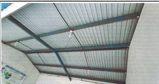
FOTO 5: Sustrucción de estructura portante de metal
