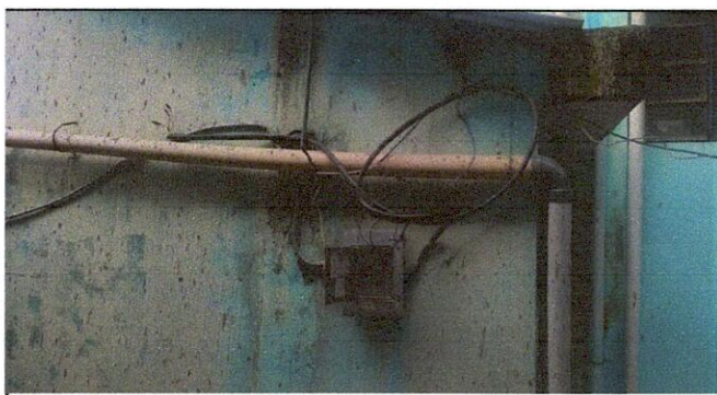
Foto 4: Se realizara la sustitución de ducto más cableado eléctrico e instalación de tablero de 8 circuitos y flípones de 50A
