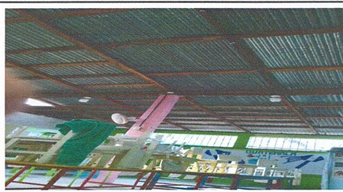
FOTO 2: Sustitución de lámina, por lámina troquelada aluzinc calibre 26, Sustitución de estructura de soporte de madera, por estructura de soporte de metal.
