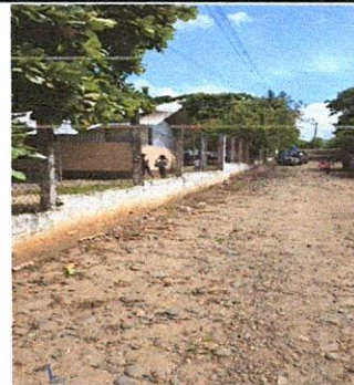
SUMINISTRO DE LEVANTADO DE BLOCK EN MURO PERIMETRAL, INCLUYE SOLERA DE CONCRETO (.15* .20*40 MTS) + 22 COLUMNAS DE CONCRETO ARMADO (.15* .20 * 3.5 MTS) + ZAPATAS (.50X.50) +
