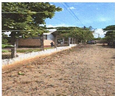
FOTO 1: SUMINISTRO DE LEVANTADO DE BLOCK EN MURO PERIMETRAL, INCLUYE SOLERA DE CONCRETO (.15* .20*40 MTS) + 22 COLUMNAS DE CONCRETO ARMADO (.15* .20 * 3.5 MTS) + ZAPATAS
