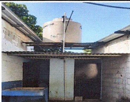
Foto 1: Sustrucción de cubierta de lámina por losa de concreto para instalación de depósito de polietileno incluye elementos de sujeción de concreto armando verticales y horizontales.
