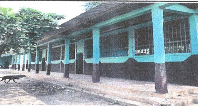
Foto 5: Sustitución de piso de concreto por piso cerámico y aplicación de pintura en muros interiores y exteriores
