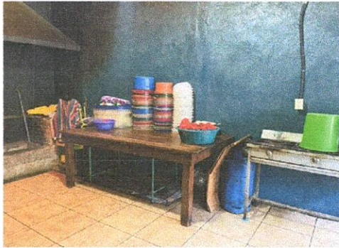
SUMINISTRO DE MUEBLE DE CONCRETO DE 2.00 MTS X 0.60 MTS REVESTIDO DE AZULEJO INCLUYE 3 DIVISIONES VERTICALES Y UNA DIVISION HORIZONTAL DE PLANCHA DE CONCRETO EN LOS
