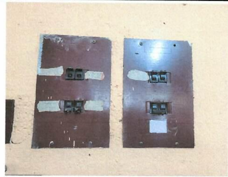
Foto 8 Caja de flipones en el interior de la dirección.
