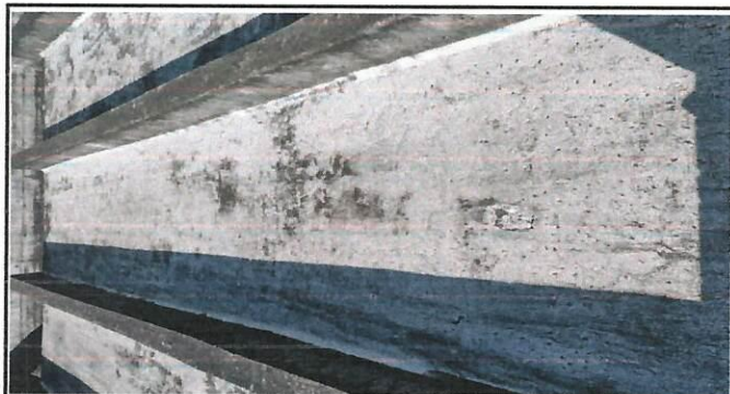
ÁREA DAÑADA EN LOSA, APLICACIÓN DE IMRERMEABILIZANTE INTEGRAL Y REPARACIÓN DE DAÑO POR EDAD DE LOSA
